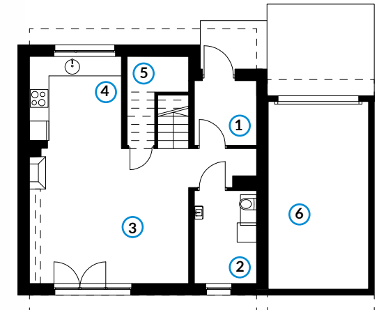
Rzut parteru
