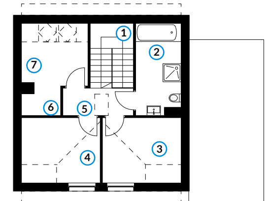
Rzut poddasza
